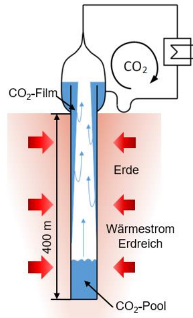
Abbildung 1: Schema der CO 2 -Sonde der U & B Wöltjen GmbH
